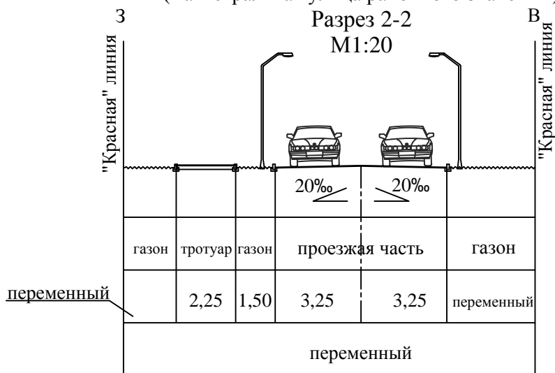
Поперечный профиль ул. Пирогова (магистральная улица районного значения)
